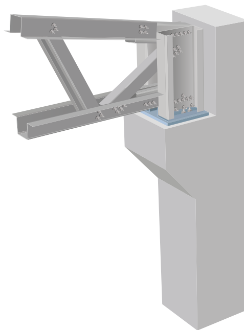
KLOUBOVÝ PŘÍPOJ NA ŽELEZOBETONOVÝ SLOUP
